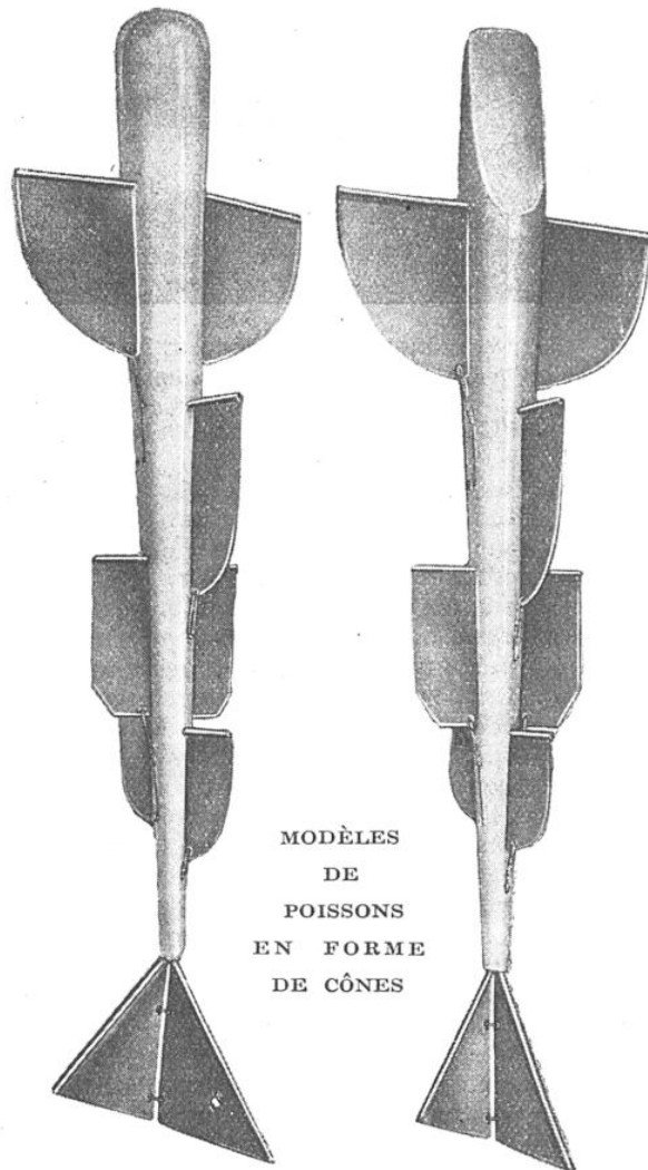
Ces deux modèles de forme allongée portent des nageoires en aluminium dont le bord antérieur, replié, est enfilé sur une tige en acier. La partie postérieure de ces appendices est rattachée par un caoutchouc à la carène de bois. En vibrant sous les remous de l'eau, les nageoires assurent la stabilité.
