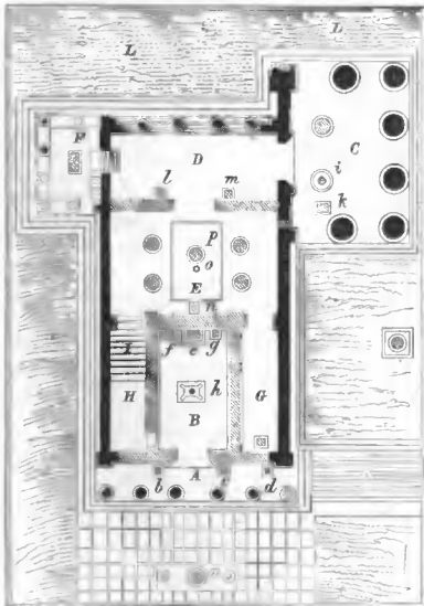
Coupe géométrale de l'Erechtheum.
