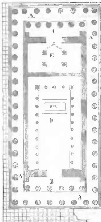
Plan géométral du Parthénon.
