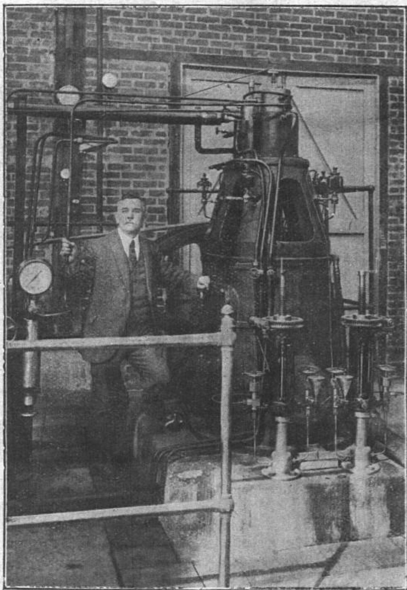
FIG. 5. — Vue d'un hypercompresseur de 700 m 3 /heure.
