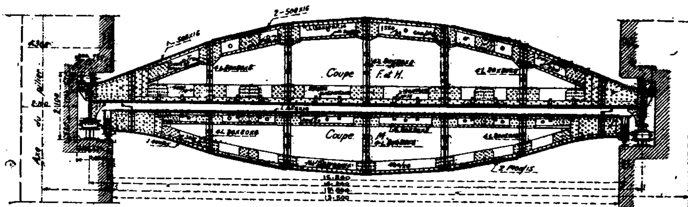
Coupe par l'axe des vannes.
