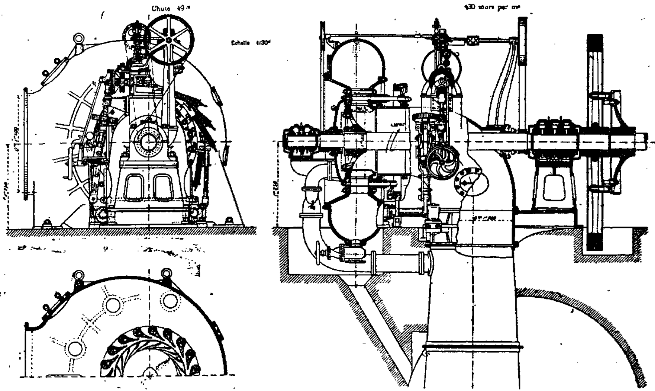
Fig. 1. — Turbine Francis de 1.600 HP, de l'usine de Saint-Gervais-les-Bains.
