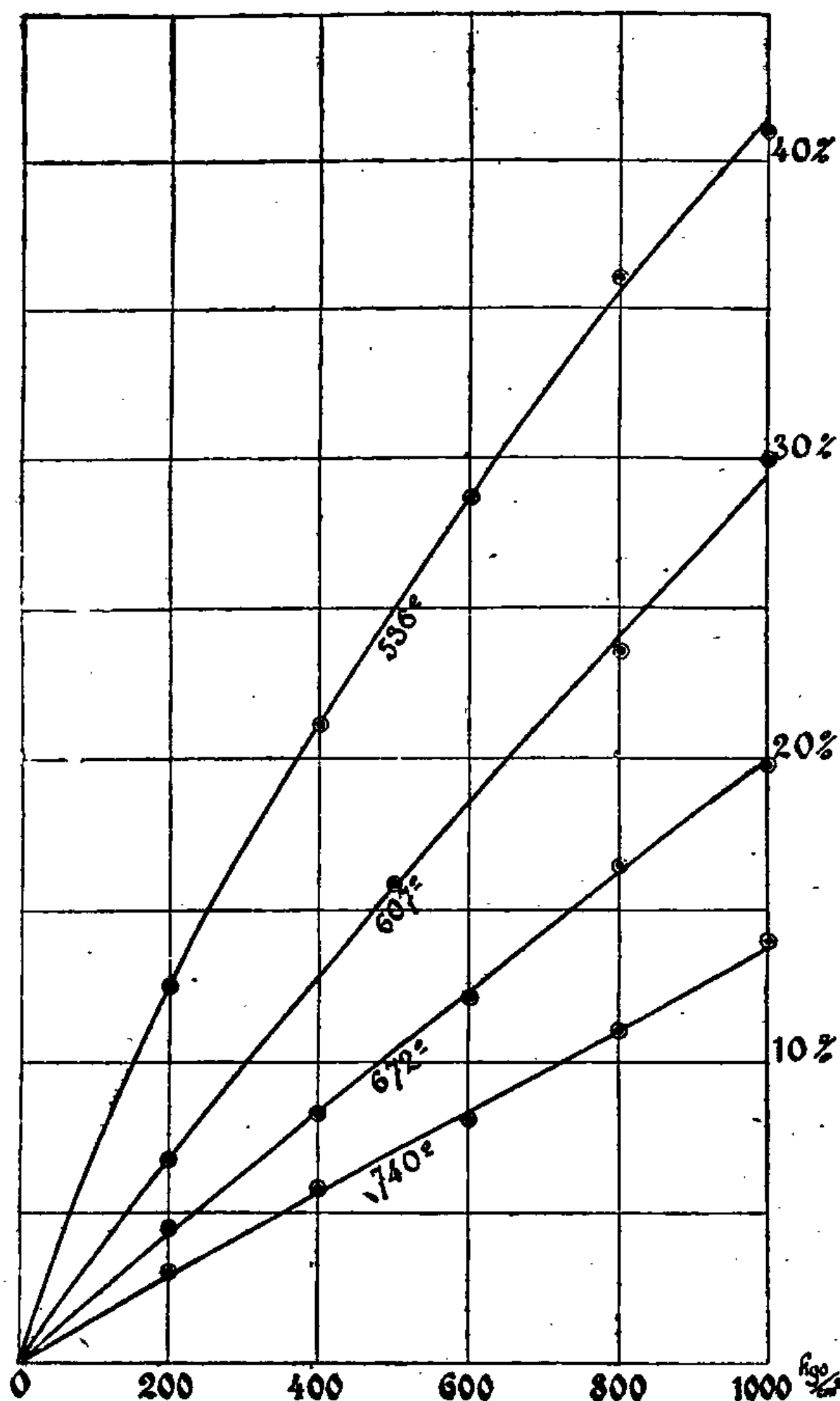
FIG. 7. — Conditions de l'équilibre jusqu'à 1.000 kg/cm².
