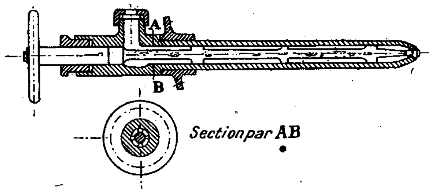
Fig. 2. — Pulvérisateur de mazout par pression. 1 er modèle (à pointeau).
