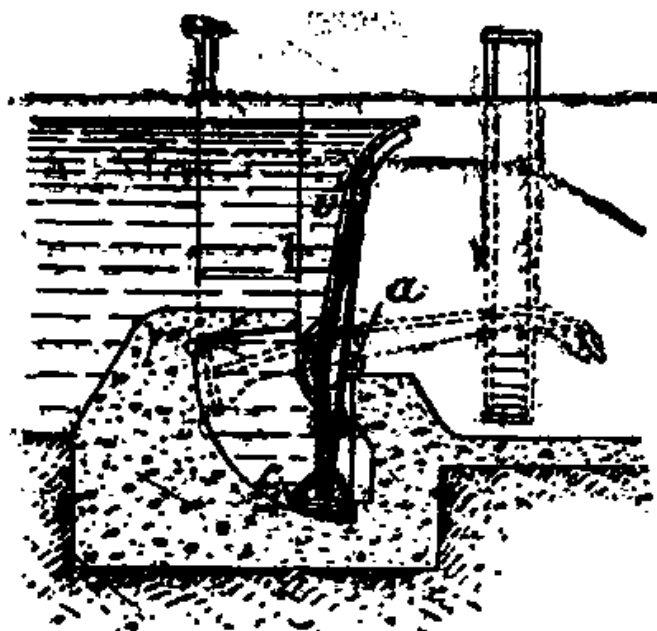
Fig. 9. — Coupe d'un barrage automatique à vanne équilibrée par en dessous, dit barrage à clapet.
