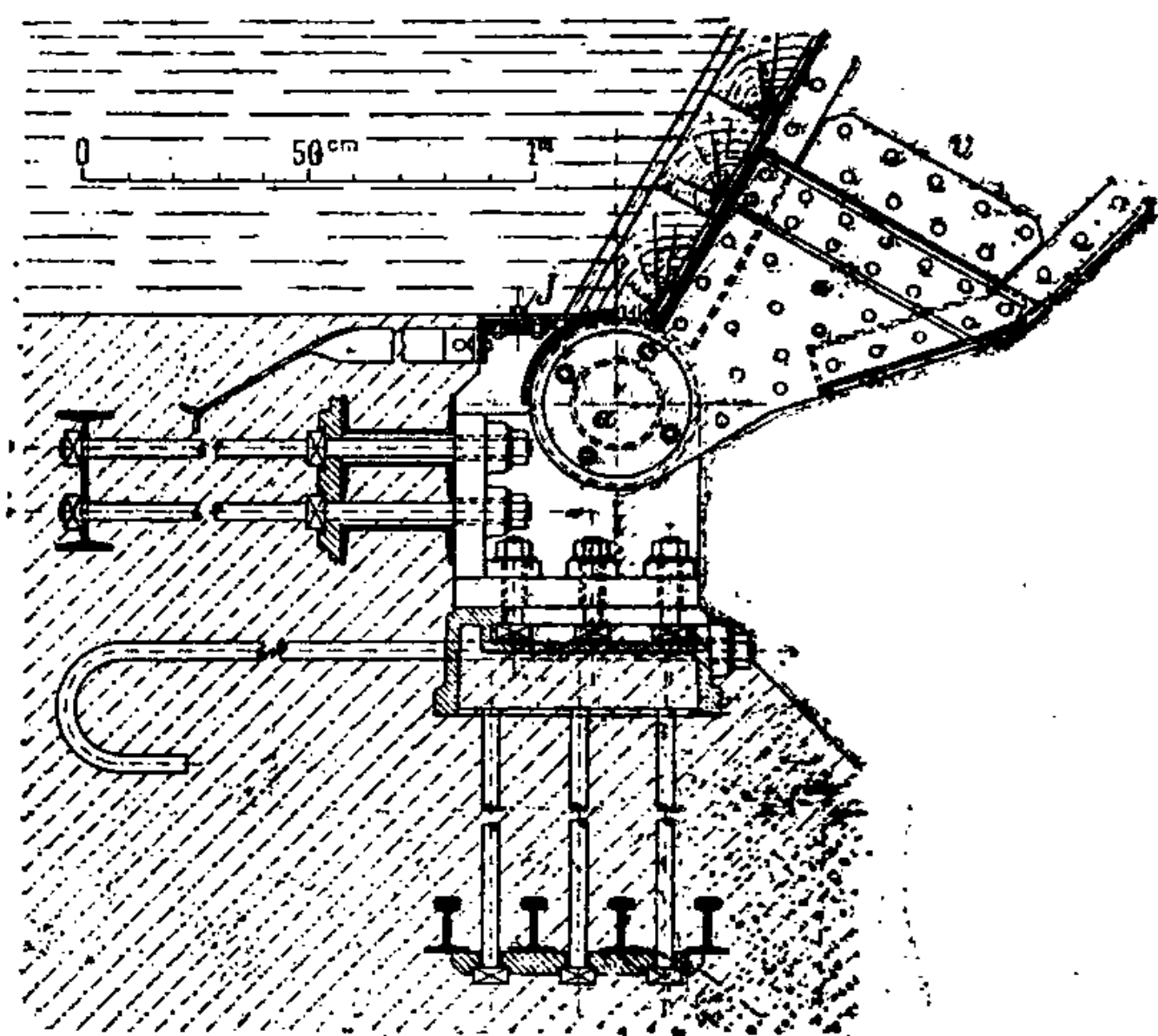
Fig. 8. — Dispositions des vannes automatiques du barrage régulateur de l'usine de Trempe.
