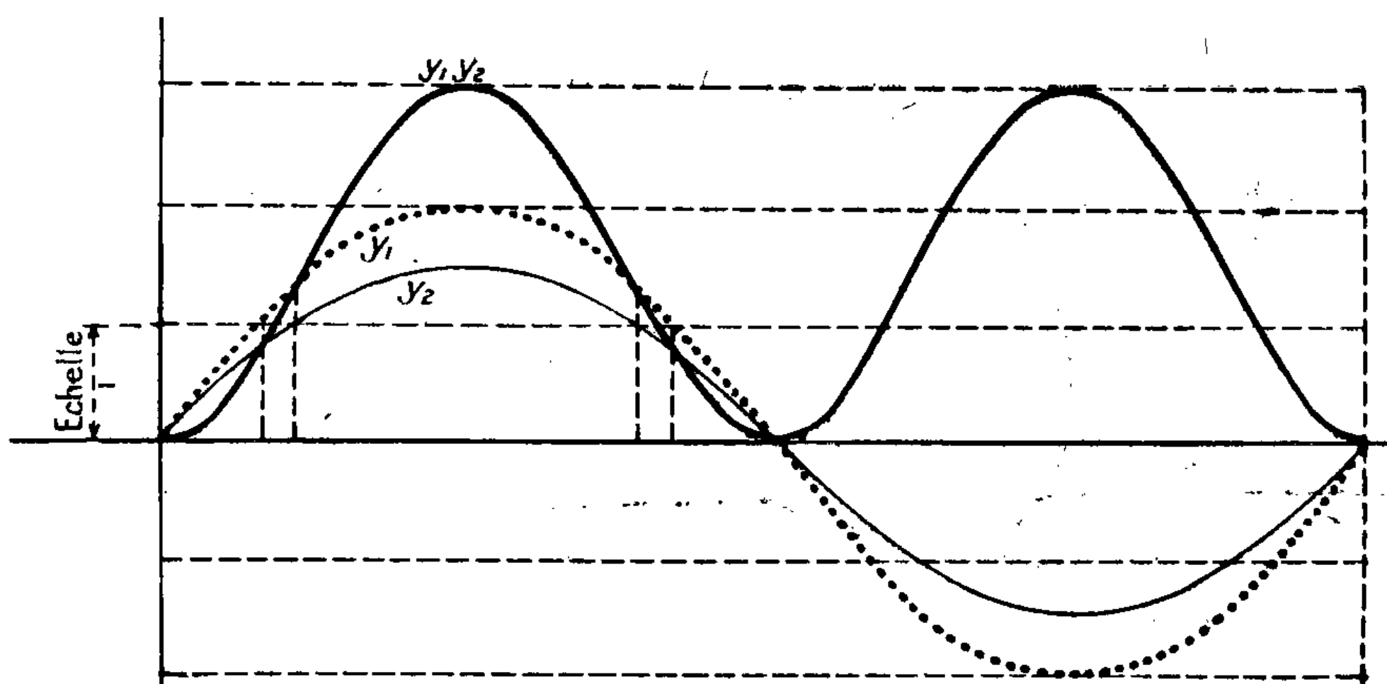
Fig. O 1 y_1 y_2 = 2 \sin \omega t \cdot 1,5 \sin \omega t .
