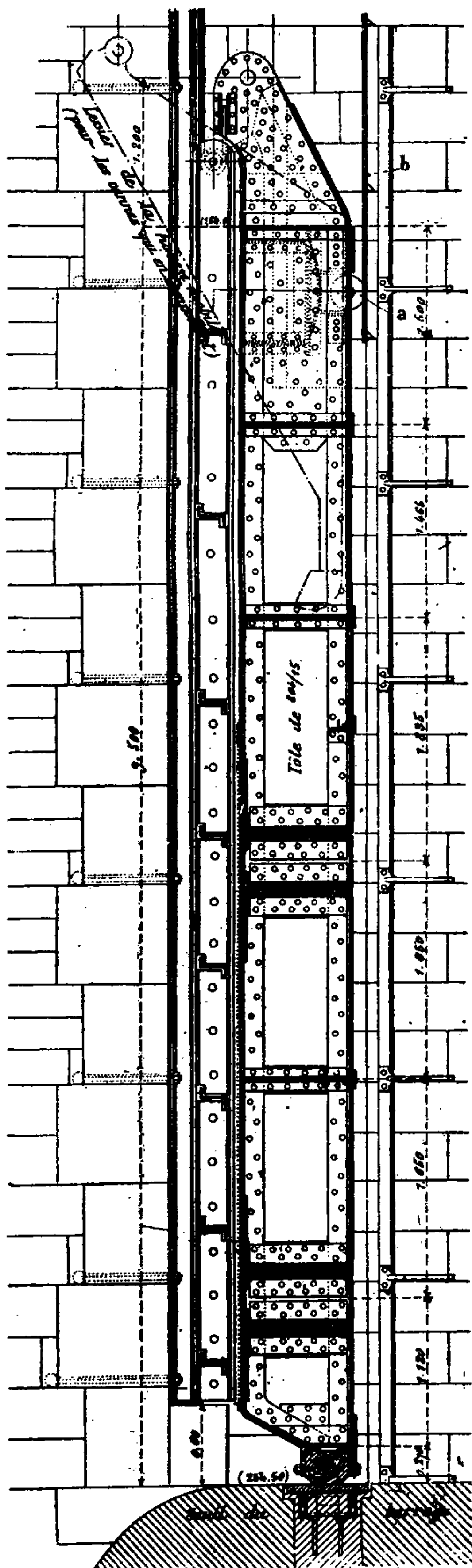
Fig. 1. — Vannes du barrage d'Augst. — Coupes verticale et horizontale.
