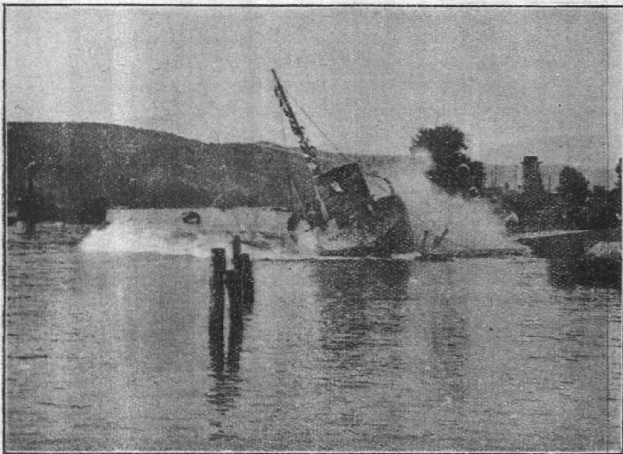
FIG. 4. — Chaland de mer de 55 mètres. Fin du lancement par le travers
