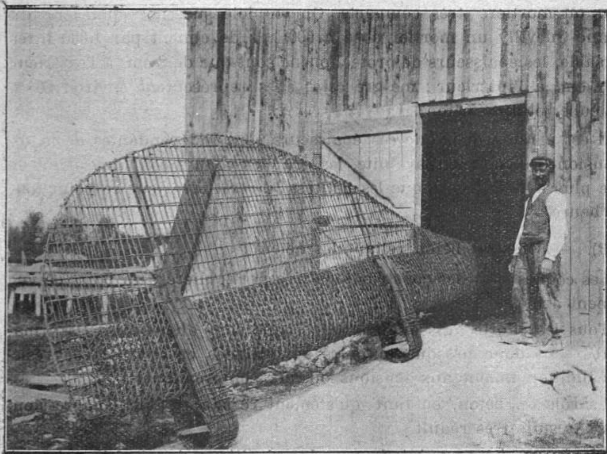
FIG. 2. — Armatures du gouvernail d'un chaland de mer en ciment armé de 55 mètres
