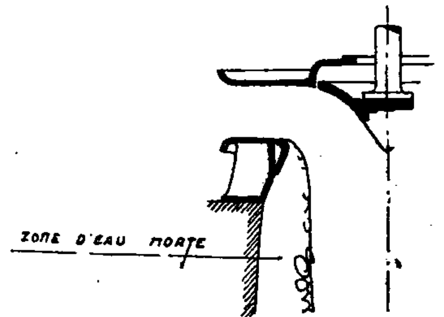
Fig. 5. — Ecoulement d'un tourbillon spiral libre dans un tube sans aube avec zone d'eau morte.
