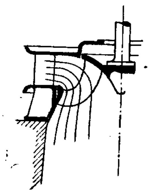
Fig. 6. — Ecoulement de l'eau en direction divergente par rapport à l'axe par suite de la présence des aubes.
