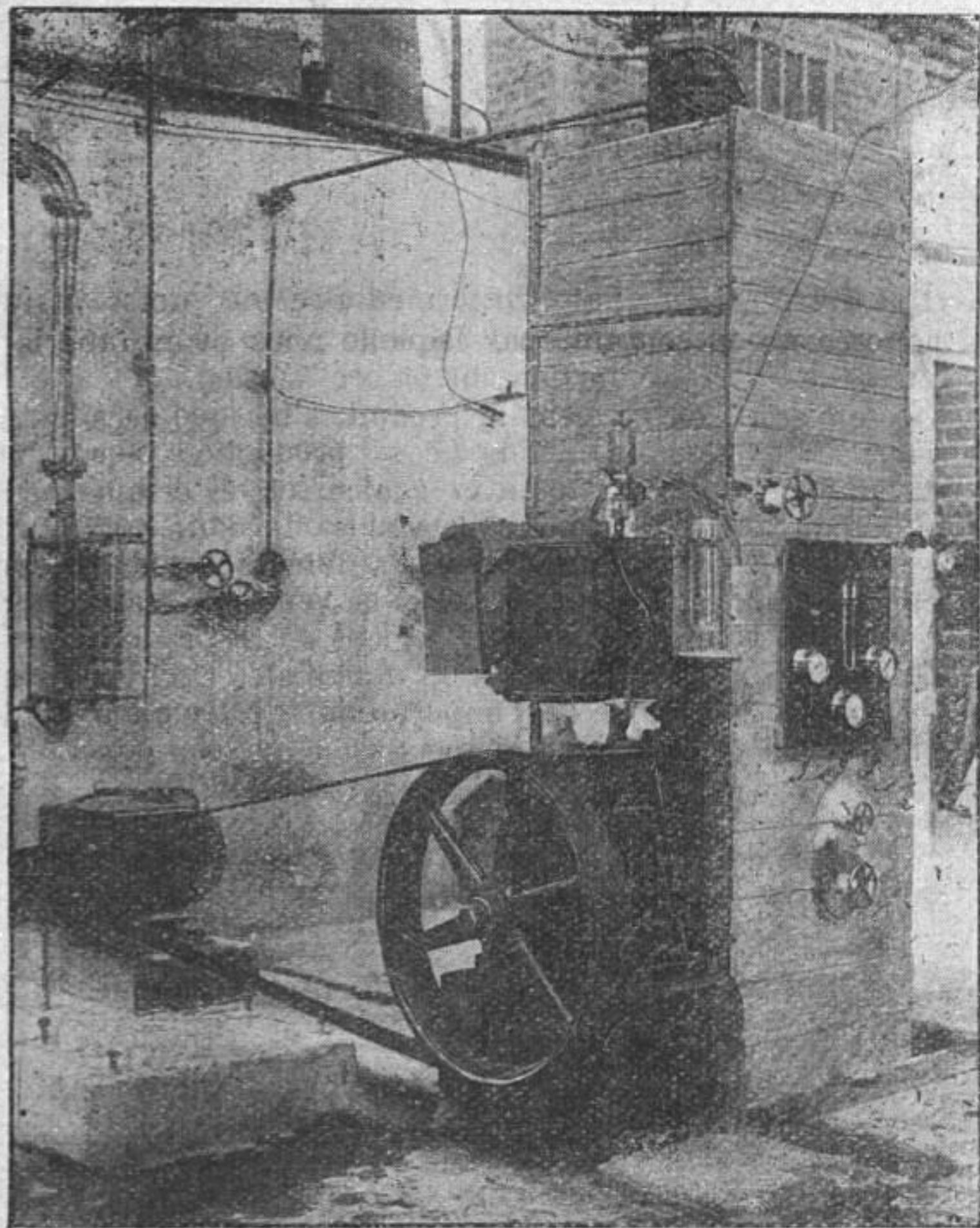
FIG. 3. — Vue d'un appareil à hydrogène de 6.000 m 3 /jour.
