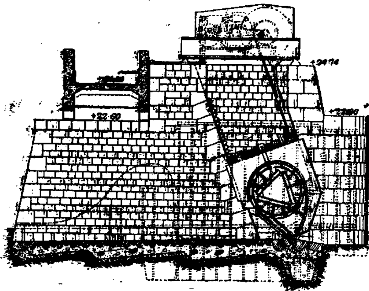
Fig. 6. — Coupe du barrage à rouleaux de l'usine d'Alfkarhely.
