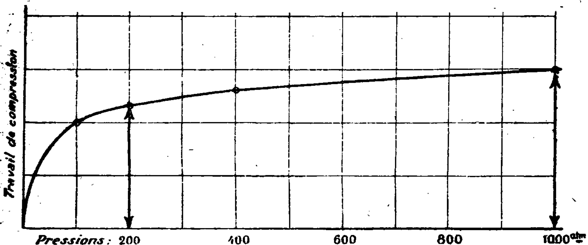
FIG. 6. — La lente variation du travail de compression avec la pression
