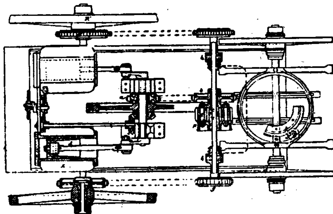
LE CHASSIS VU EN PLAN
