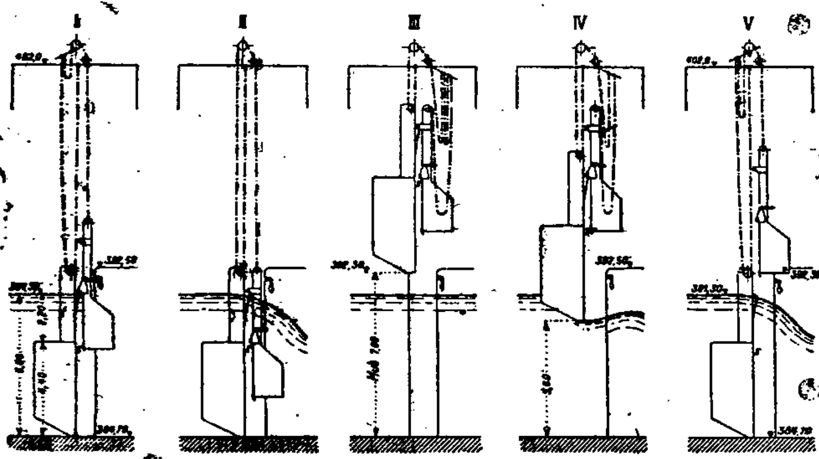
Fig. 2. — Schéma des positions successives des vannes de l'usine de Gösgen.
