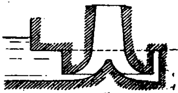
Fig. 11. — Disposition schématique d'un tube d'aspiration avec hydraucône et diffuseur à disques.
