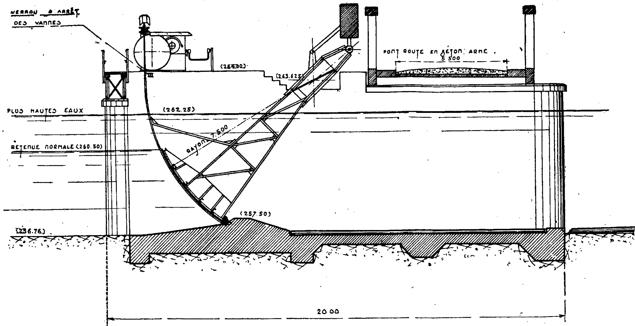
Fig. 7. — Coupe d'une vanne à secteur de l'usine du Drac-Romanche.
