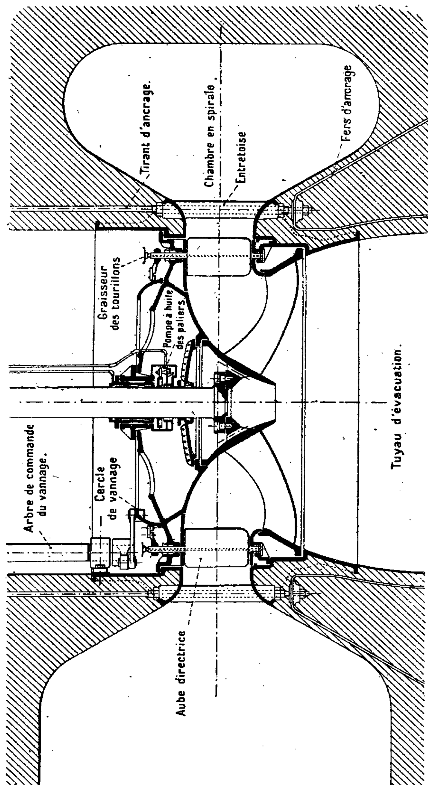
Fig. 8. — Coupe d'une turbine à grande vitesse Piccard-Pictet.
