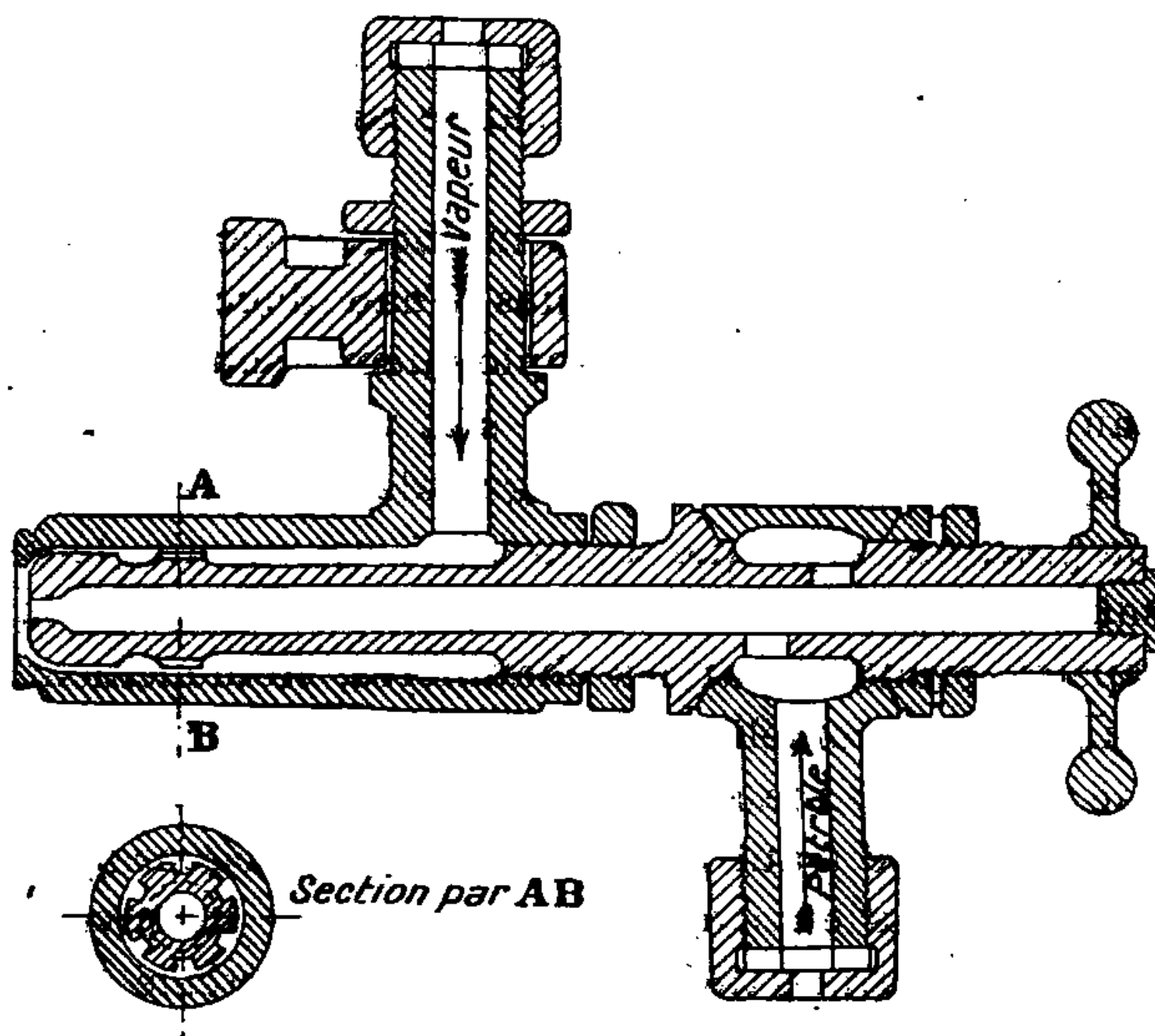
Fig. 1. — Pulvérisateur de pétrole par la vapeur, 1 er modèle (Pulvérisateur russe Choukopp).
