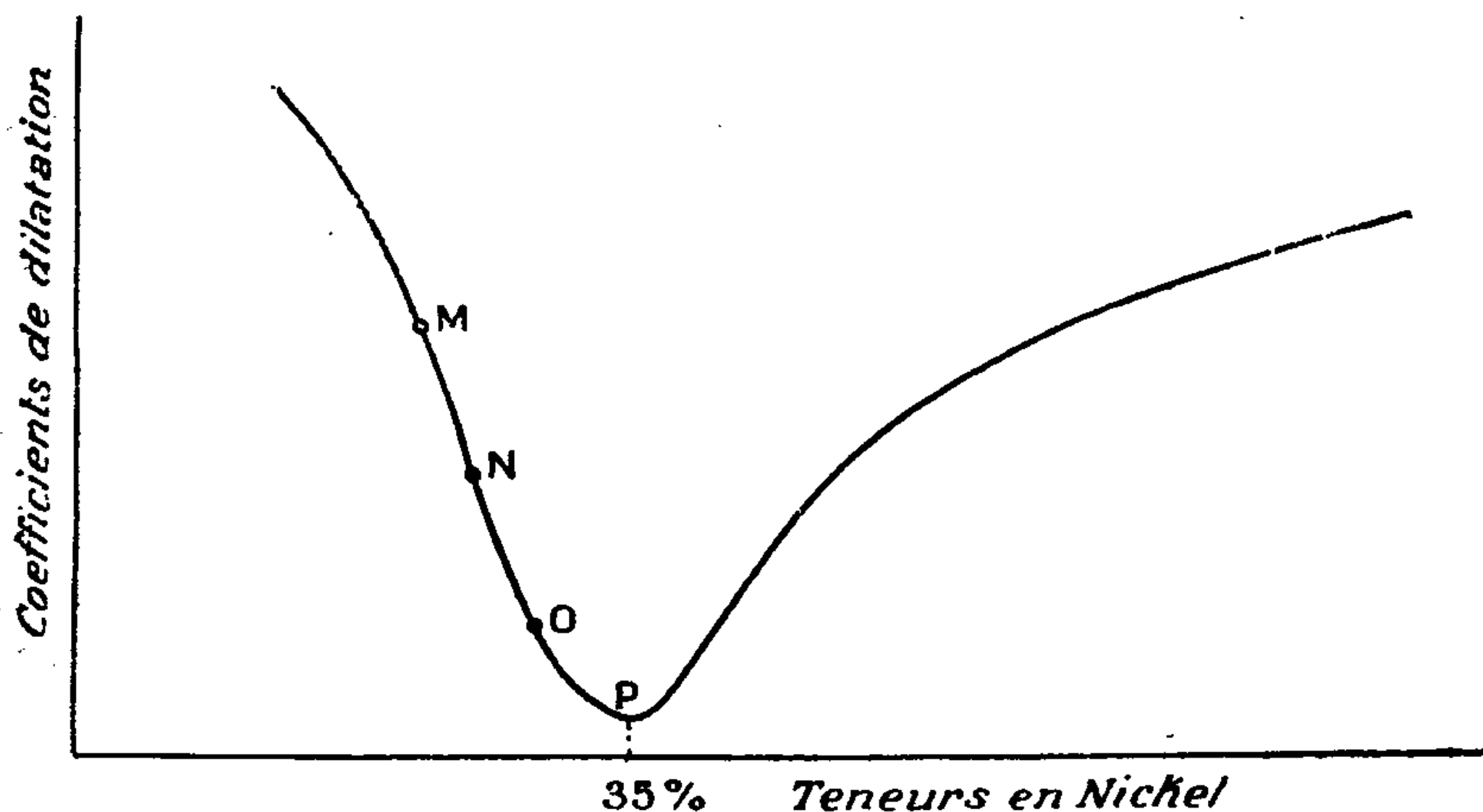
FIG. 1. — Courbe représentative de l'anomalie des aciers au nickel.
