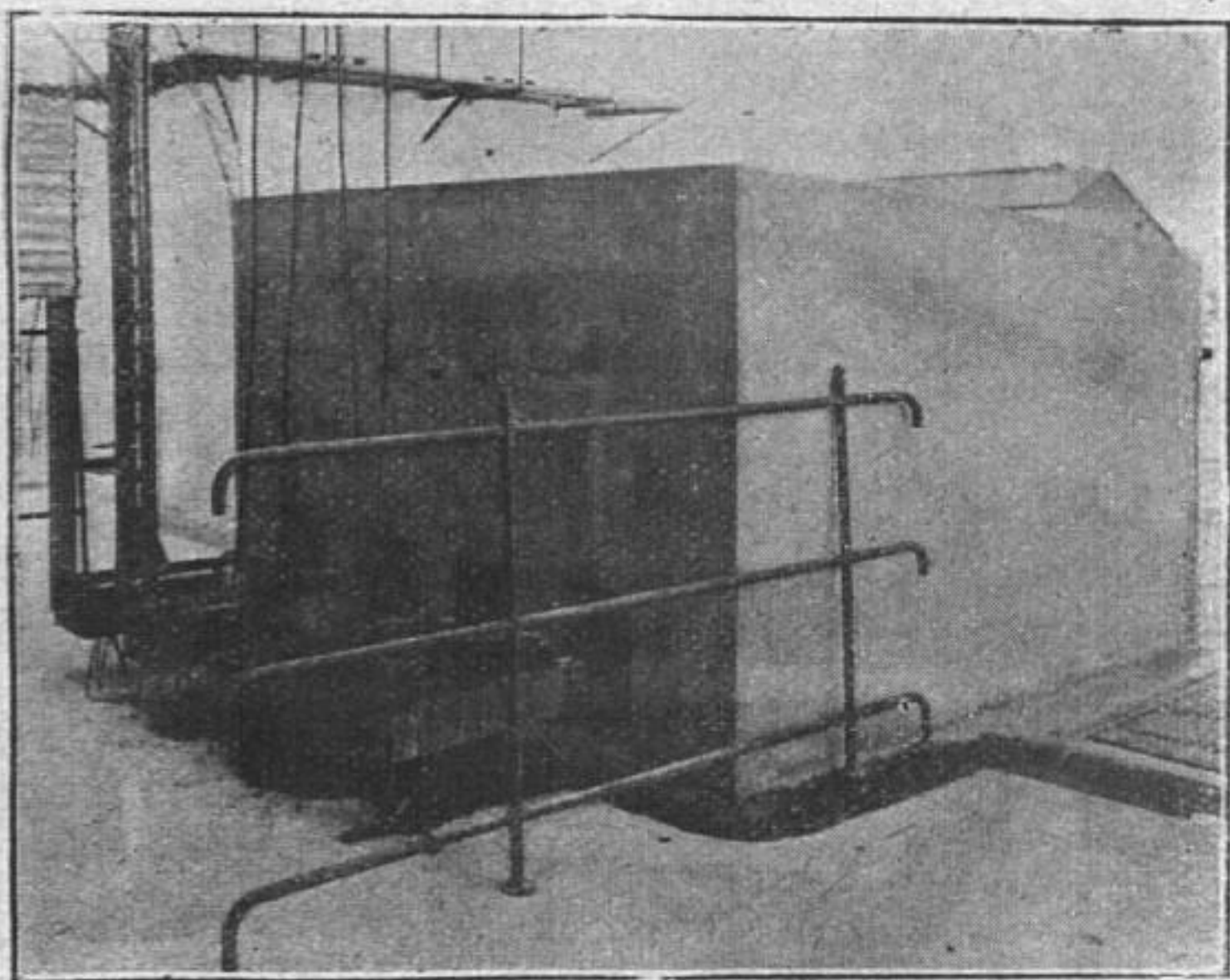
FIG. 8. — En avant, petit blockhaus contenant les 4 tubes catalyseurs horizontaux d'une installation de 1,25 t d'NH 3 p. j. En arrière, blockhaus renfermant 2 des 4 tubes d'une installation de 5 t d'NH 3 p. j.
