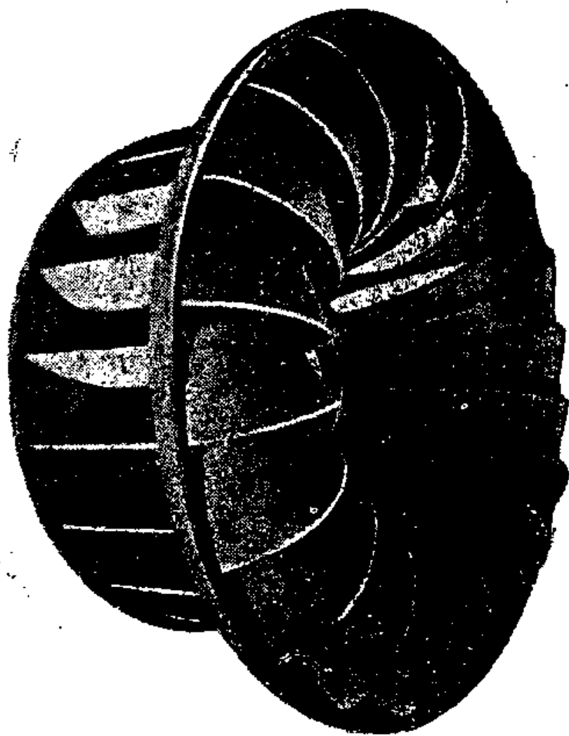
Fig. 2. — Roue mobile de turbine Francis à nombre de tours spécifique élevé.
