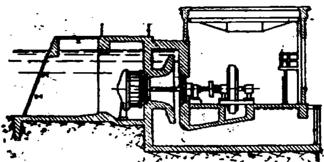
Fig. 10. — Turbine montée avec diffuseur à disques à la sortie.
