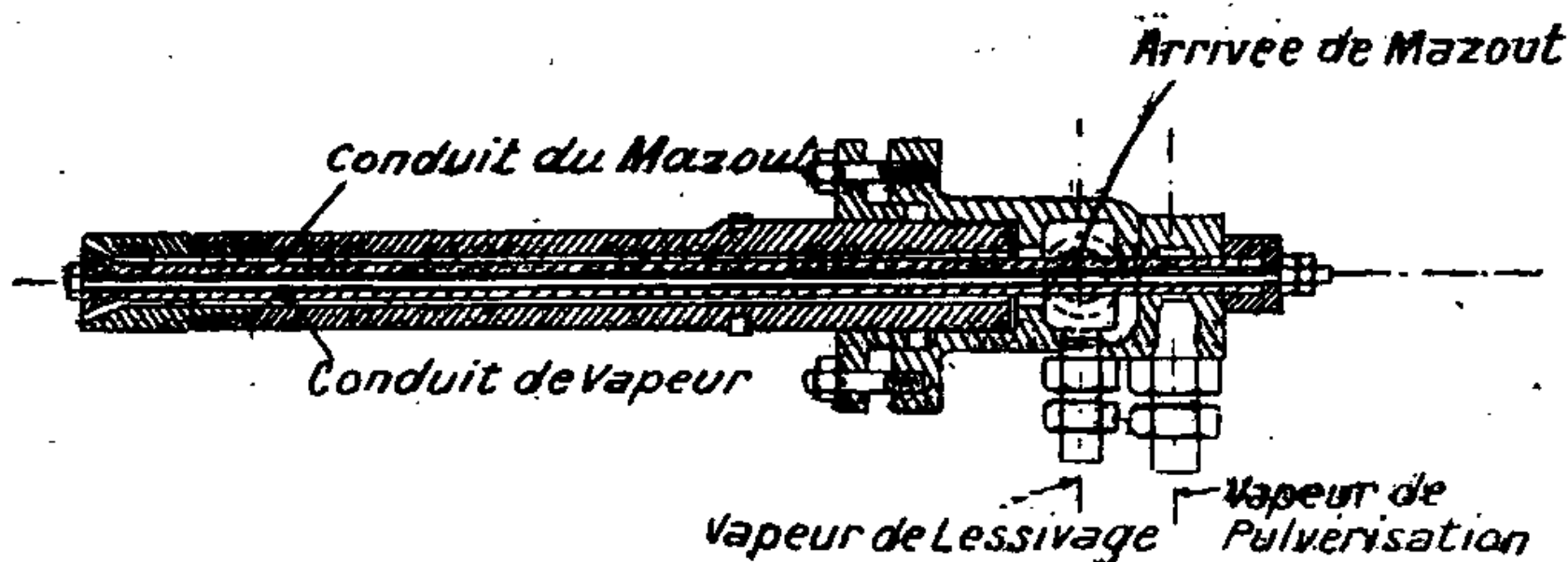
Fig. 1 bis. — Pulvérisateur de mazout par la vapeur ou l'air comprimé. Système Walsend-Howden. — 2 e modèle (plus récent).
