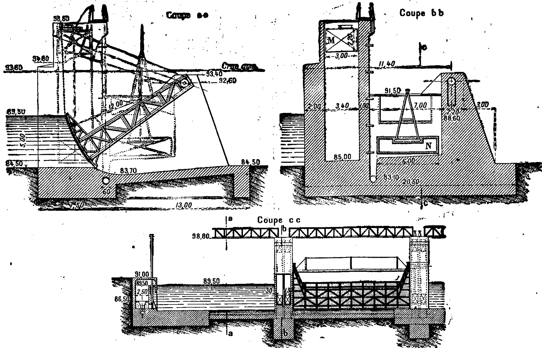
Fig. 10. — Coupe d'un barrage automatique sur fleuve avec effacement par-dessus
