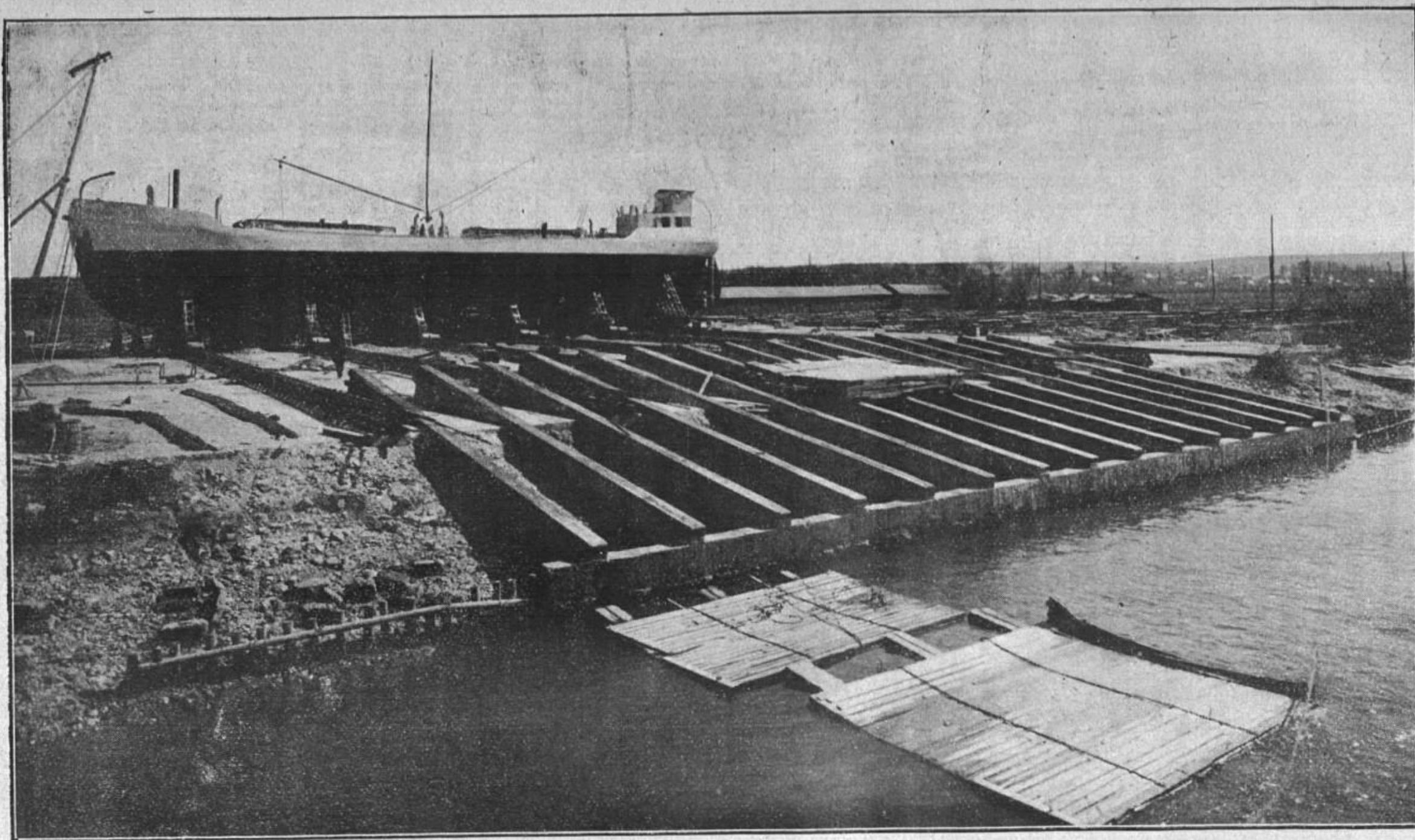
FIG. 1. — Chaland de mer en ciment armé. Longueur : 55 mètres. Port en lourd : 1.350 tonnes. Avant son transport sur la cale de lancement par le travers. Au premier plan : glissière en béton de la cale de lancement
