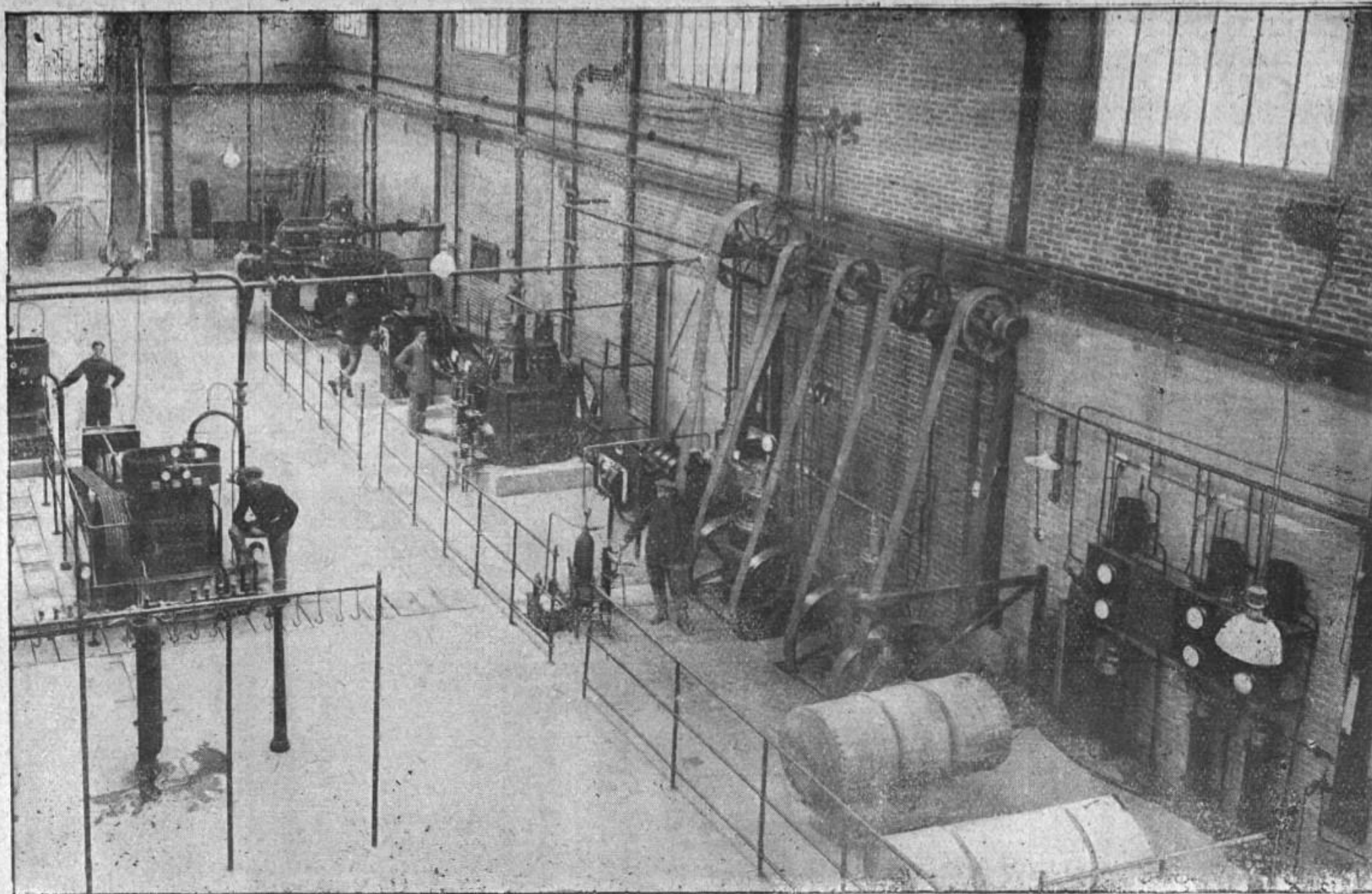
FIG. 10. — Vue d'ensemble de la salle de compression et de l'installation d'extraction de l'ammoniaque. Au fond, l'appareil à azote.
