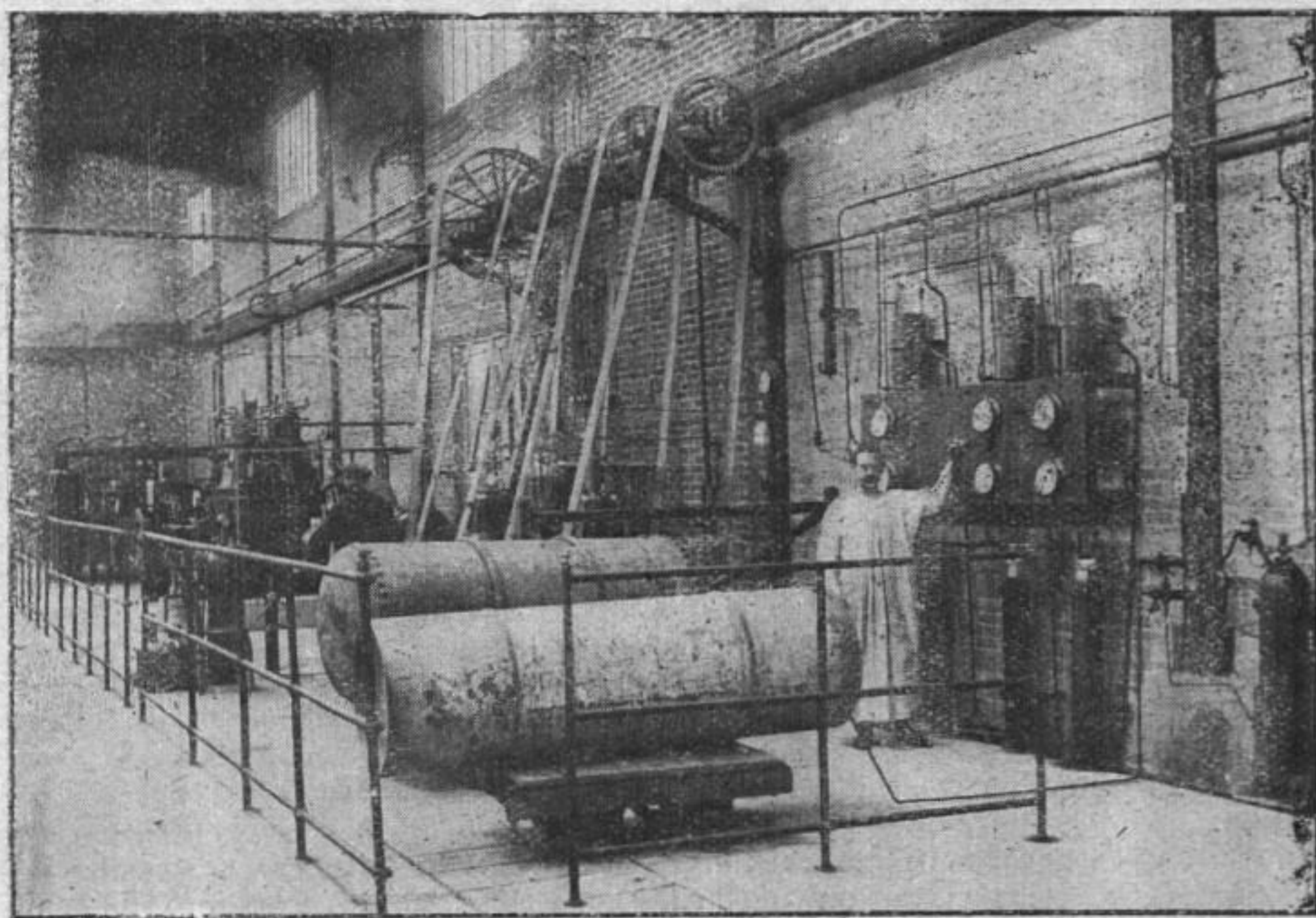
FIG. 9. — Vue des appareils de condensation, d'extraction et d'emménagement de l'ammoniaque à l'usine de Montereau.
