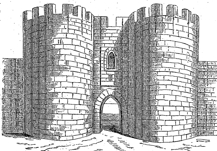
213. — PORTE D'AIGUES-MORTES.
